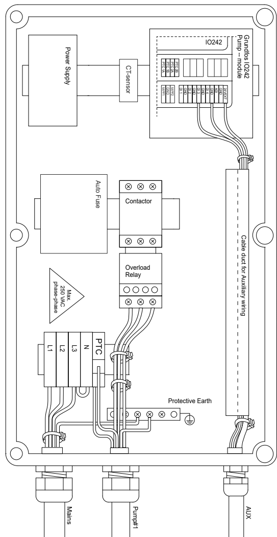
Трифазні з'єднання для одного насоса без нейтралі, лише для Норвегії
