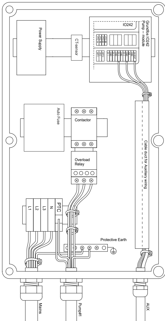
Трифазні з'єднання для одного насоса
